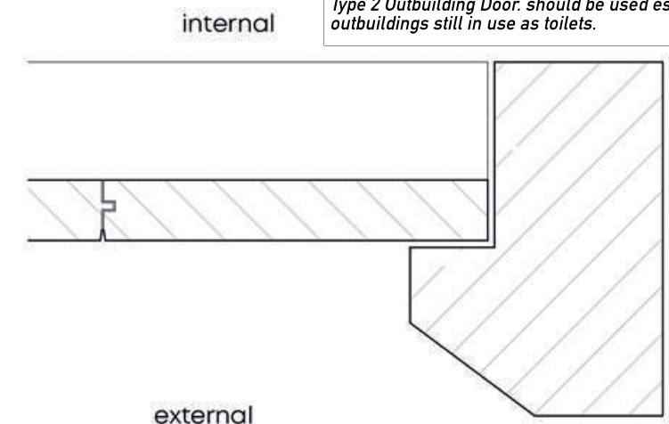
Door and Frame Section 1:2
