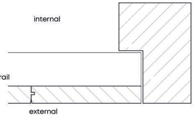
Door and Frame Section 1:2
